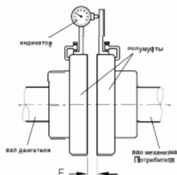
Рис. 4 Схема измерения аксиальной несоосности (непараллельности осей)
